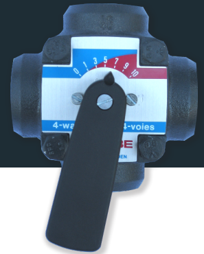
4-putni miješajući ventil
